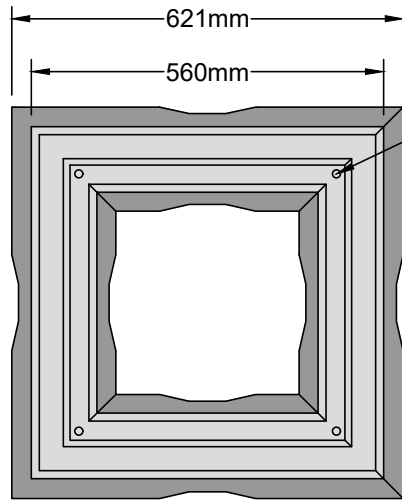
VUE DE DESSUS DU NTS
