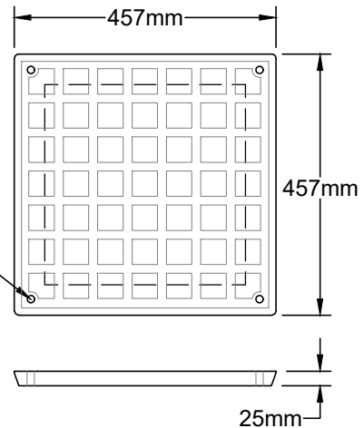
DETAIL DE LA PLAQUE D'ADAPTATION NTS
