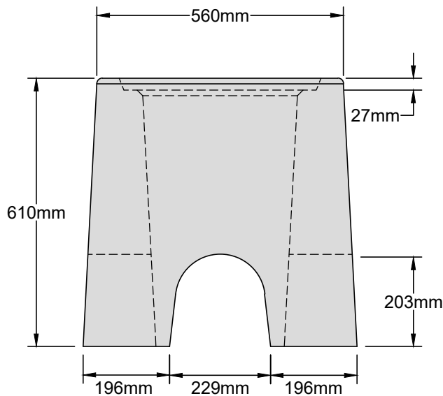
VUE LATÉRAL DU NTS
